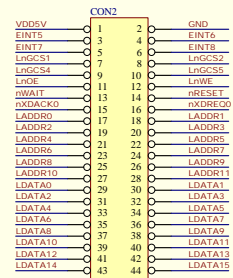
HEADER 22X2
